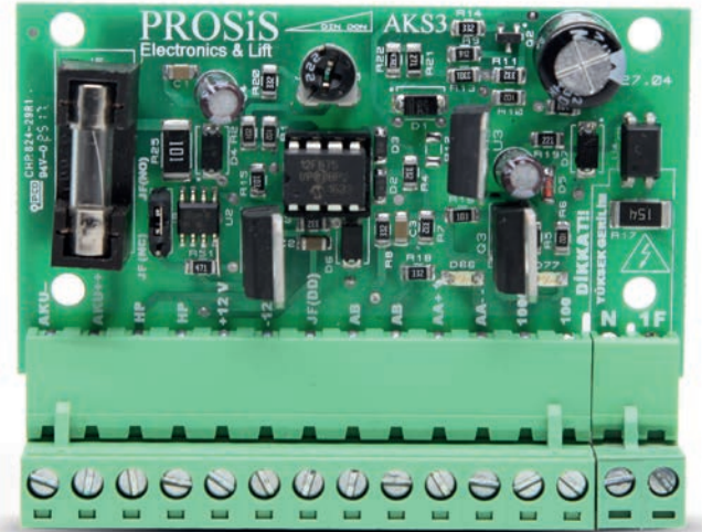
AKS 3 Revizyon Kartı AKS 3 Revision Card
